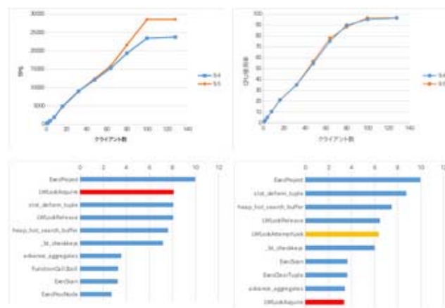
定点観測(スケールアップ検証・参照系)の結果
