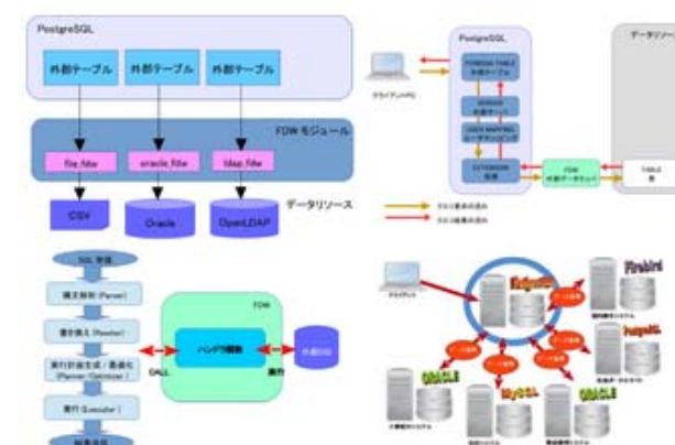
FDW(外部データラップ)概要図
