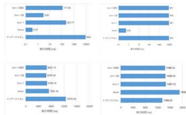
BRIN Index検証の結果
